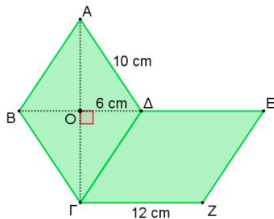
AB\Gamma\Delta ρόμβος \Gamma\Delta ΕΖ παραλληλόγραμμο
