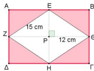
AB\Gamma\Delta ορθογώνιο E\Theta HΖ ρόμβος
